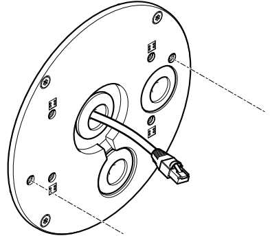
AXIS P33-VE
