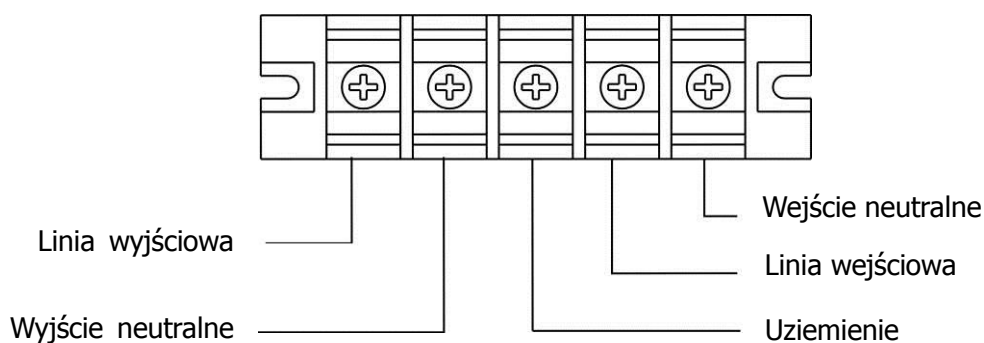
Blokowy schemat połączeń terminalu
