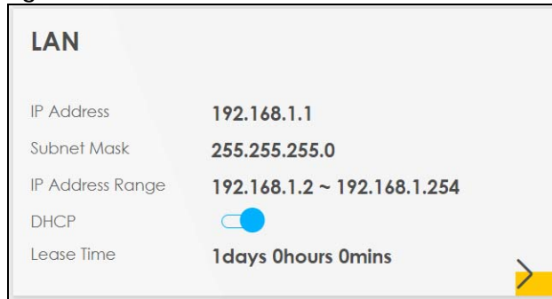
Figure 60 LAN
