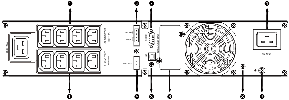
3000VA Tylny panel standardowego panelu
