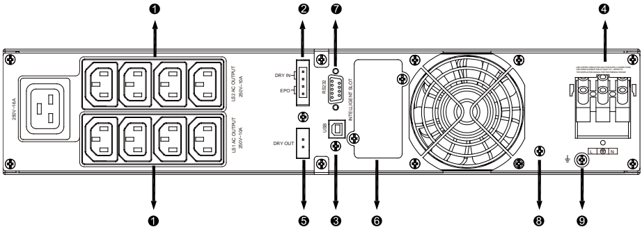
3000VA Tylny panel super-ładowanego modelu
