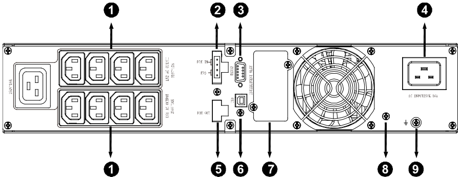
3000VA Tylny panel standardowego panelu
