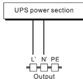
Schemat połączenia
