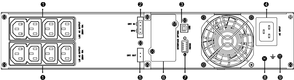
2000VA Tylny panel super-ladownego modelu
