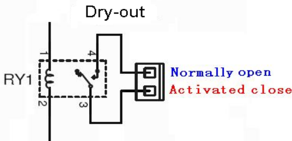
Schemat podłączenia wyjściowego styku beznapięciowego
