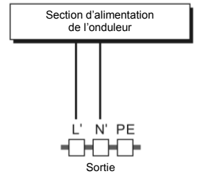
Schéma de connexion
