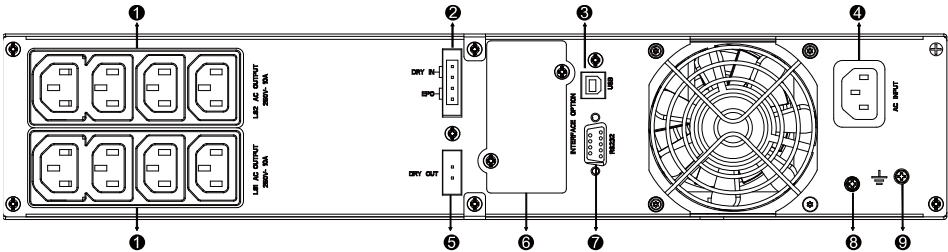
Tylny panel standardowych 1000VA /1500VA/2000VA & 1000VA /1500VA super-ladownych modeli
