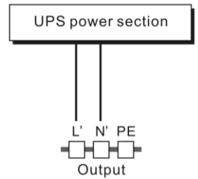
Anschlussdiagramm
