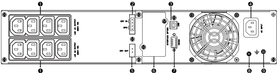
1000VA / 1500VA / 2000VA Standard & 1000VA / 1500VA Supercharger-Modell, Rückseite
