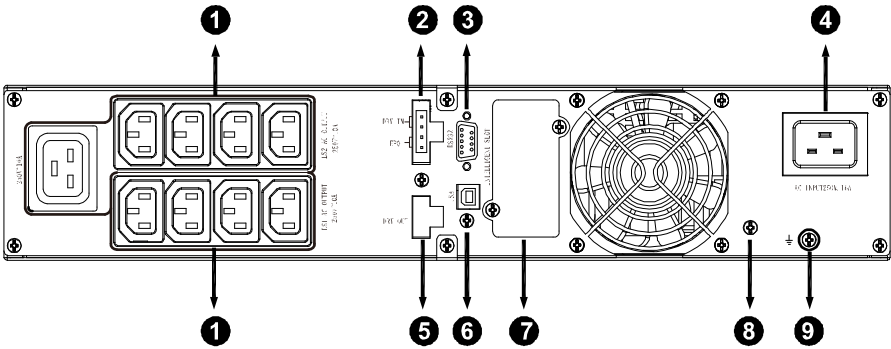
Panneau arrière pour modèle 3000 VA standard
