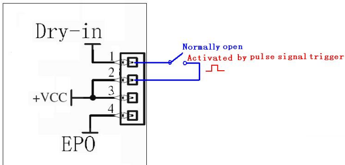
Schemat podłączenia wejściowego styku beznapięciowego
